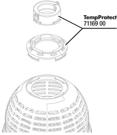
JBL TempProtect II askı seti
