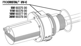
JBL PC UV-C elektrik birimi
