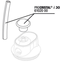
JBL PC i30 hortum 4/6+ hava giriş kapağı
