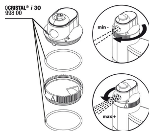
JBL PC i30 scarico con regolazione
