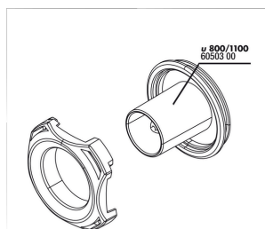
JBL PF "u" copertura+ raccordo tubi flessibili
