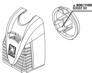
JBL PF "u" grata protettiva + regolazione
