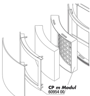
JBL CP m greenline attacco modulo FilterPad
