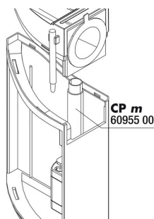
JBL CP m greenline tubo d'uscita
