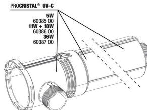
PROCRISTAL® UV-C 5W 60385 00 11W + 18W 60386 00 36W 60387 00 JBL PC UV-C 5 W Kit de carcaça, 2 peças
