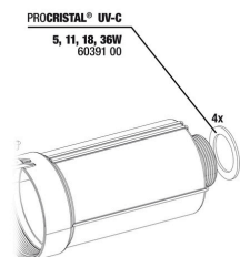
PROCRISTAL® UV-C 5, 11, 18, 36W 60391 00 JBL PC UV-C Vedações ligação de mangueira
