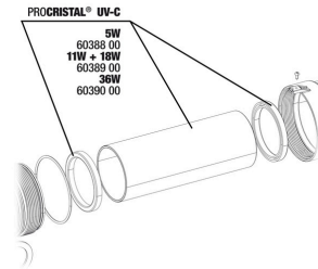
PROCRISTAL® UV-C 5W 60388 00 11W + 18W 60389 00 36W 60390 00 JBL PC UV-C Kit invólucro de vidro+ refletor
