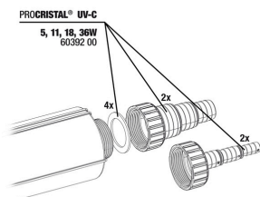
PROCRISTAL® UV-C 5, 11, 18, 36W 60392 00 JBL PC UV-C Kit ligação de mangueira
