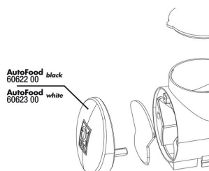
JBL AutoFood Suporte completo, 1 kit
