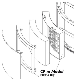
JBL CP m greenline Suporte módulo FilterPad
