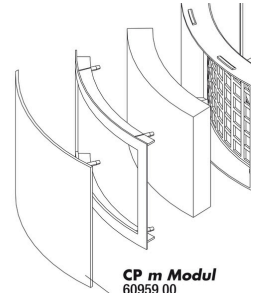
JBL CP m greenline Tapa de manutenção Módulo
