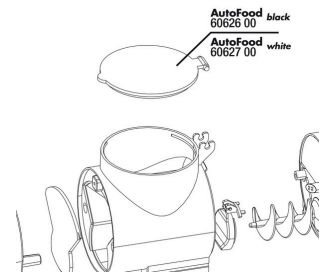
JBL AutoFood Deksel
