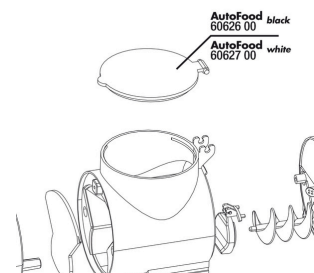
JBL AutoFood Deckel Futterkammer
