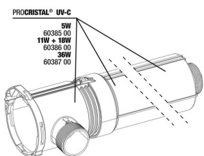
JBL PC UV-C 5 Вт корпус в компл., 2 части
