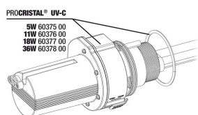
JBL PC UV-C электроблок
