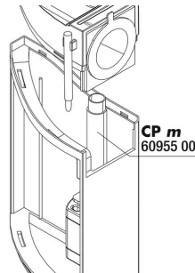
JBL CP m greenline outlet pipe
