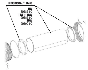
JBL PC UV-C kit cilindro vetro+riflettore
