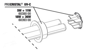
JBL PC UV-C kit protezione bruciatore
