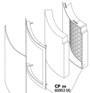
JBL CP m greenline sostegno FilterPad
