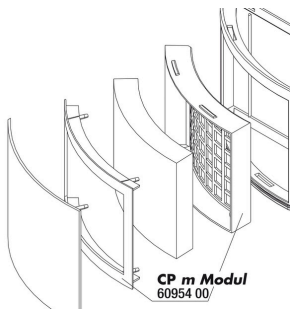
JBL CP m greenline Fixation module FilterPad
