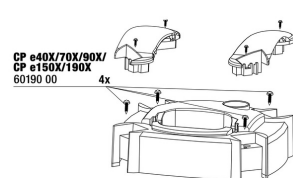
JBL CP e4/7/9/15/1900/1,2 винты для головы помпы
