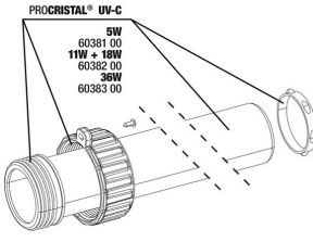
JBL PC UV-C kuvars cam piston seti
