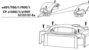
e401/700/1/900/1 CP e1500/1/e1901 60189 00 4x JBL CP e4/7/9/15/1900/1/2 tutacak vidaları
