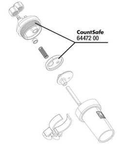
JBL CO2 Count Safe conta plakası
