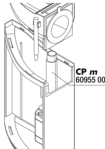
JBL CP m greenline Auslaufrohr
