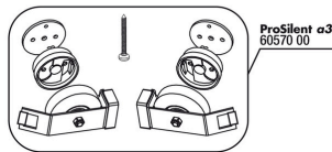
JBL PS set membrane a100-a400
