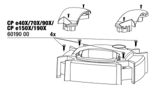
JBL CP e4/7/9/15/1900/1,2 Parafusos cabeça bomba
