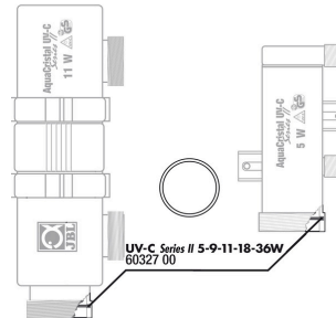
JBL AC UV-C 5,9,11 W Junta tórica, carça
