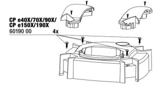
CP e4/7/9/15/1900/1 CP e1500/1900 60190 00 4x JBL CP e4/7/9/15/1900/1,2 PK vidaları
