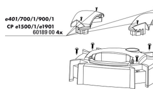
JBL CP e4/7/9/15/1900/1/2 handle screws
